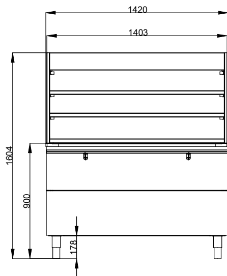
Zepředu
